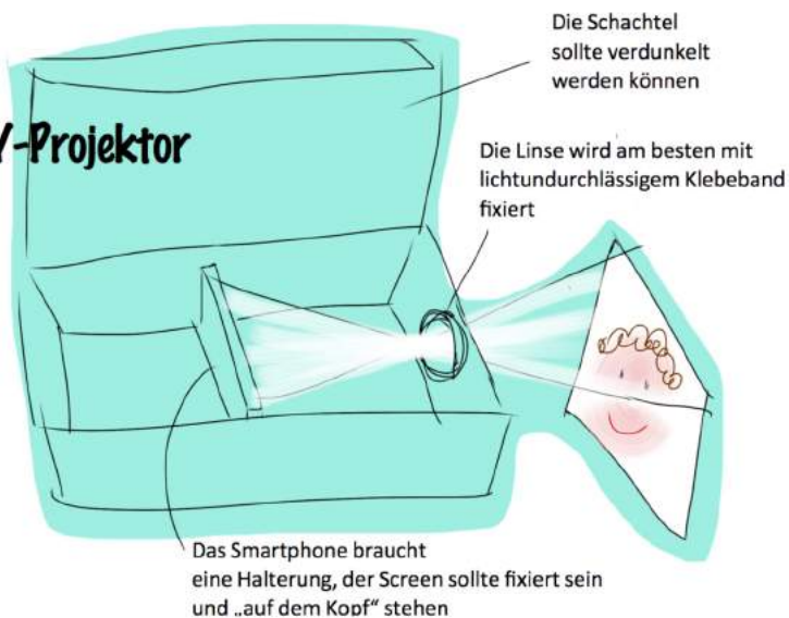
Bauplan eines Projektors (Skizze)
