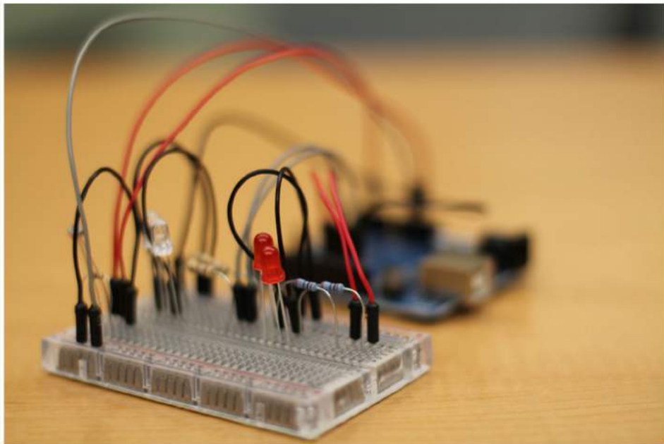
Steckplatte mit Arduino (im Hintergrund) – Foto: CC BY Betsy Weber, URL: https://www.flickr.com/photos/betsyweber/5849382494/ ; URL zur Lizenz: https://creativecommons.org/licenses/by/2.0/
